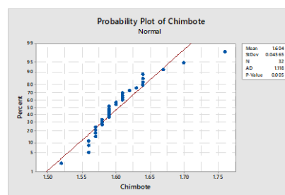
(f) Gráfico de probabilidad normal del Nivel superficial del mar de la estación de Chimbote. 1984-2015.
