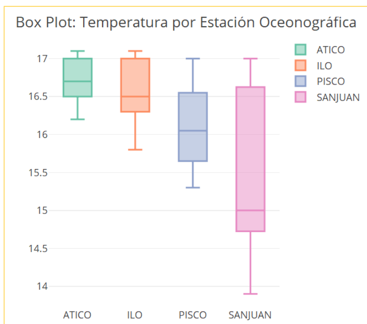
Figura 76. Boxplot 9e la temperatura por estación oceanográfica: Crucero Oceanográfico Sur - del 27 julio al 10 agosto 2014.
