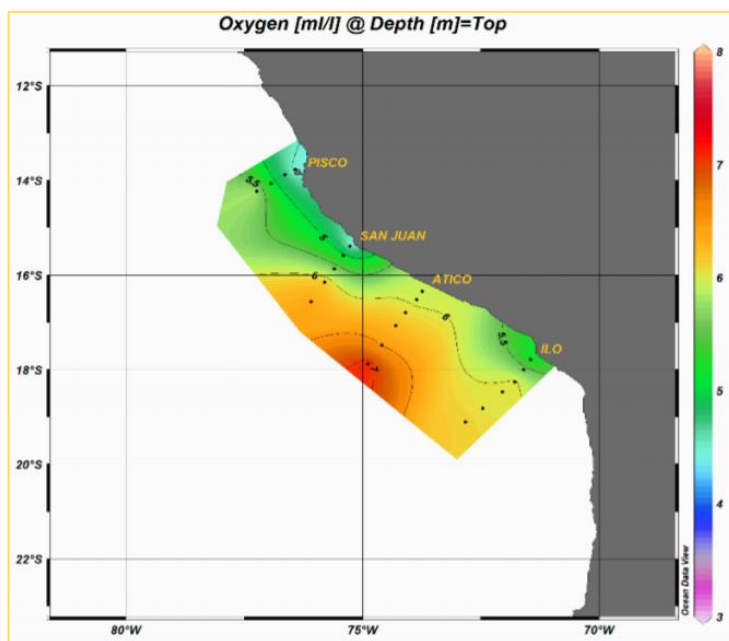
Figura 71. Registro del oxígeno por estación oceanográfica: Crucero Oceanográfico Sur - del 27 julio al 10 agosto 2014.
