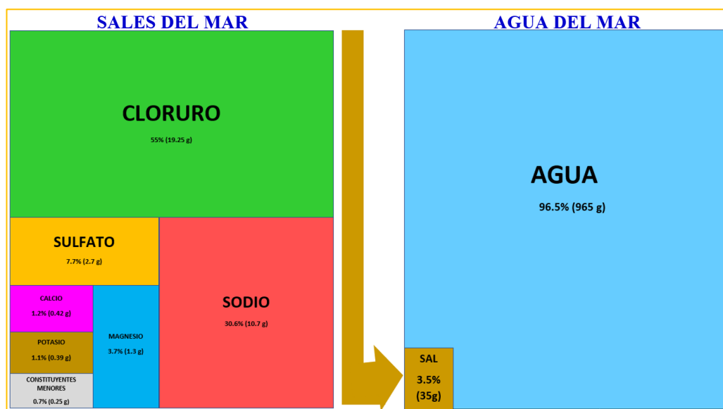
Figura 4. Composición química del agua de mar.
