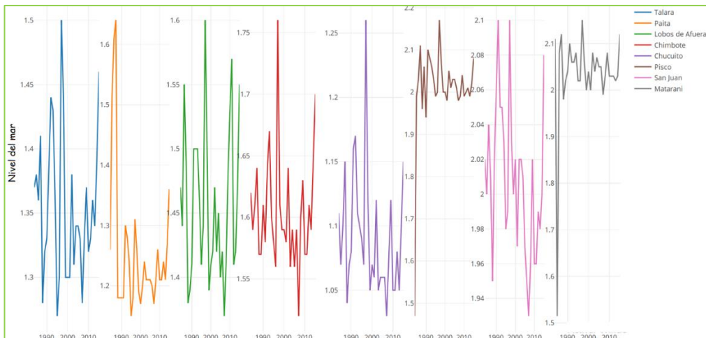
Figura 7A. Secuencia de las medias de los niveles superficiales del mar en las estaciones de Chucuito, Paita, Talara, Lobos de Afuera, Pisco Chimbote, San Juan y Matarani. 1984-2015.
