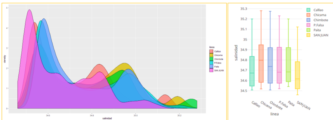
Figura 57. (a) Función de densidad empírica de la salinidad en las líneas de monitoreo en estudio. (b) Boxplot de la salinidad en las líneas de monitoreo en estudio. Las líneas de monitoreo corresponden al Callao, Chicama, Chimbote, P.Falsa, Paita y San Juan respectivamente.
