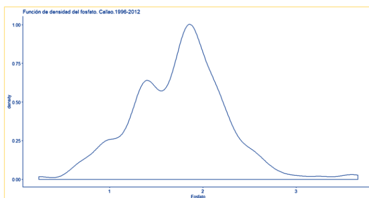
Figura 11A. Función de densidad empírica de la variable fosfato.
