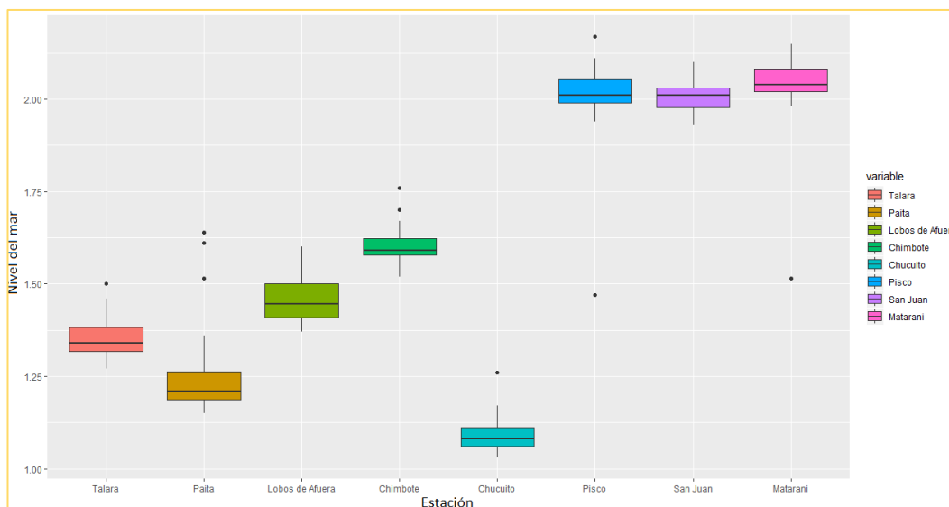
Figura 18. Distribución espacial del nivel superficial del mar por estaciones de monitoreo. 1984- 2015.
