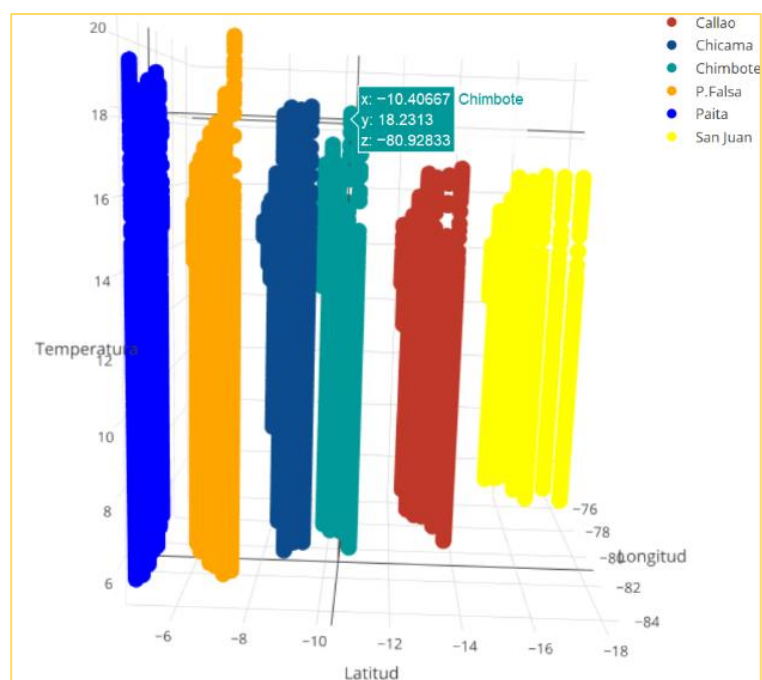
Figura 55. Distribución de la temperatura de acuerdo con la longitud y latitud según las líneas de monitoreo: Callao, Chicama, Chicbote, P. Falsa, Paita y San Juan.
