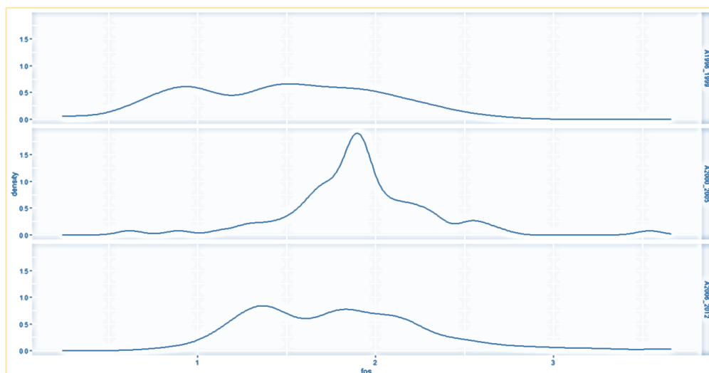
Figura 15A. Función de densidad empírica del fosfato por periodos de tiempo: 1996-1999, 2000-2005, 2006-2012
