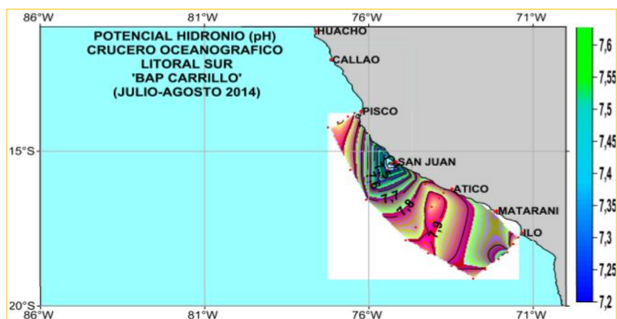
Figura 79. Registro del pH por estación oceanográfica: Crucero Oceanográfico Sur - del 27 julio al 10 agosto 2014.
