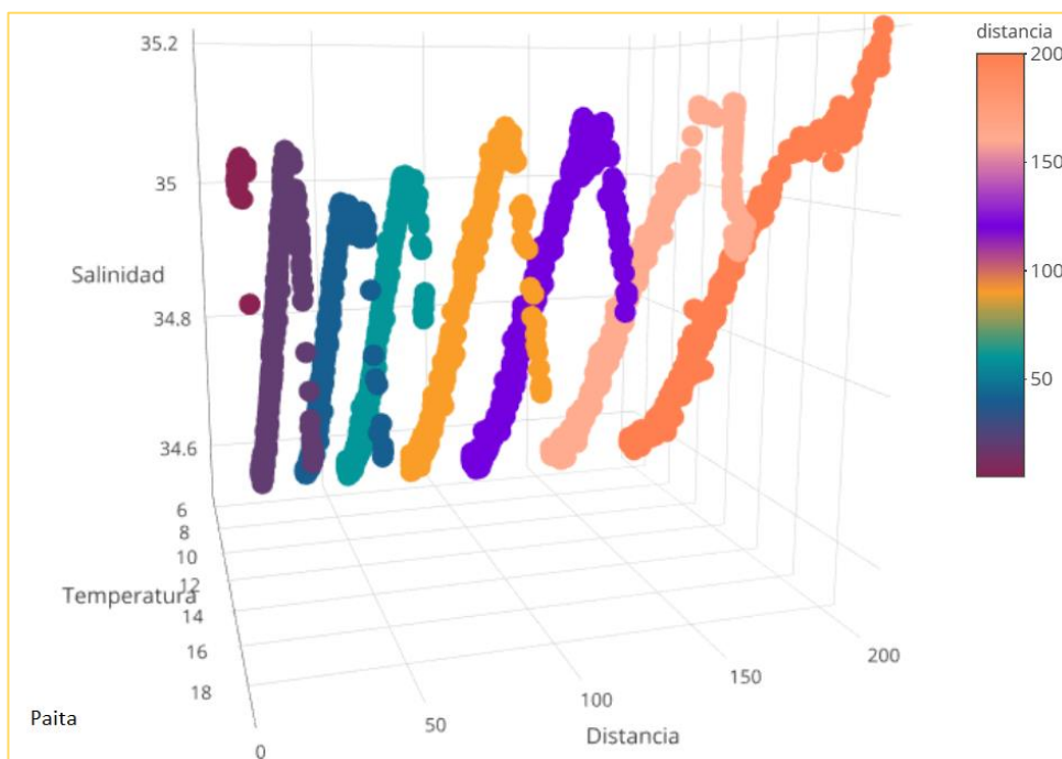
Figura 53A. Distribución conjunta de la temperatura y salinidad de acuerdo con la distancia en Paita.
