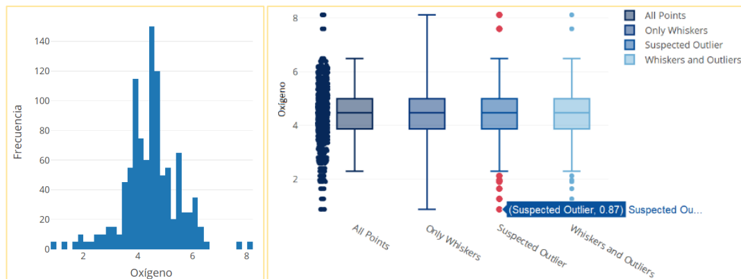
Figura 38. Histograma y boxplot de la variable oxígeno. Callao 1996-2012.
