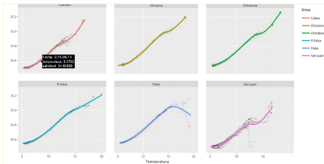
Figura 40A. Distribución conjunta de la temperatura y salinidad de acuerdo las líneas de monitoreo: Callao, Chicama, Chimbote, P. Falsa, Paíta y San Juan.
