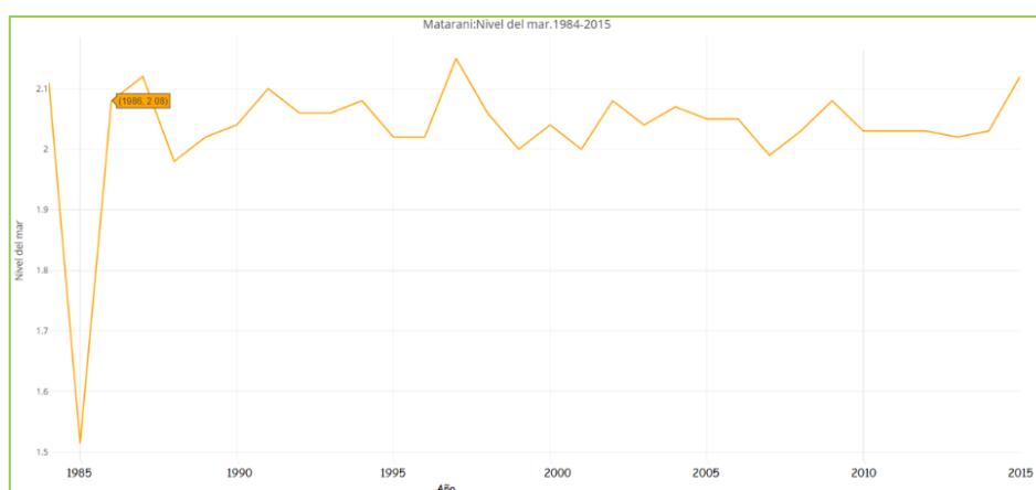
Figura 6A. Dinámica del nivel superficial del mar en la estación de Matarani.
