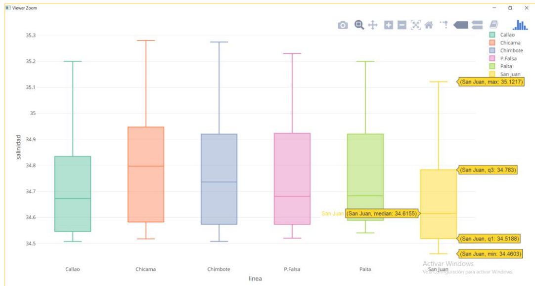
Figura 58. Diagrama de cajas de la salinidad en el Callao, Chicama, Chimbote, P. Falsa, Paíta y San Juan respectivamente.
