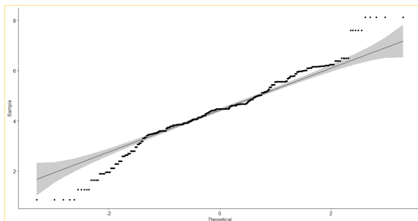
Figura 40. Q-Q plot. de la variable oxígeno.
