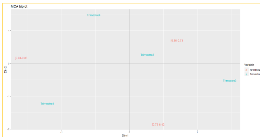
Figura 37A. Biplot: Visualización de la correspondencia entre las categorías de la variable nitrito y los trimestres del año.
