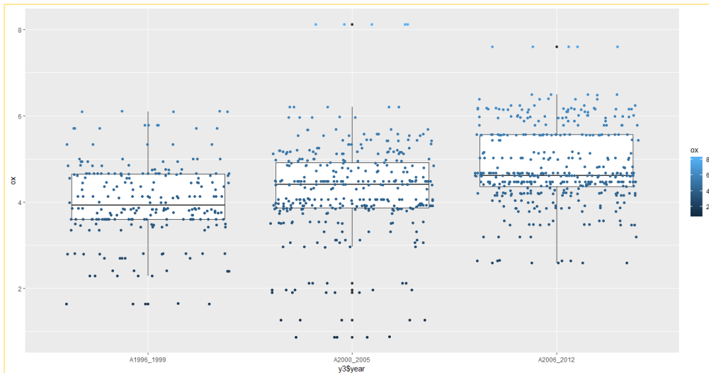
Figura 42. Evolución del oxígeno por periodos de tiempo: 1996-1999, 2000-2005, 2006-2012.
