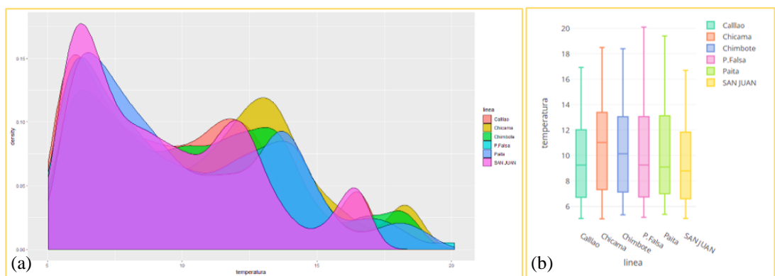
Figura 53. (a) Función de densidad empírica de la temperatura en las líneas de monitoreo en estudio. (b) Boxplot de la temperatura en las líneas de monitoreo en estudio.
