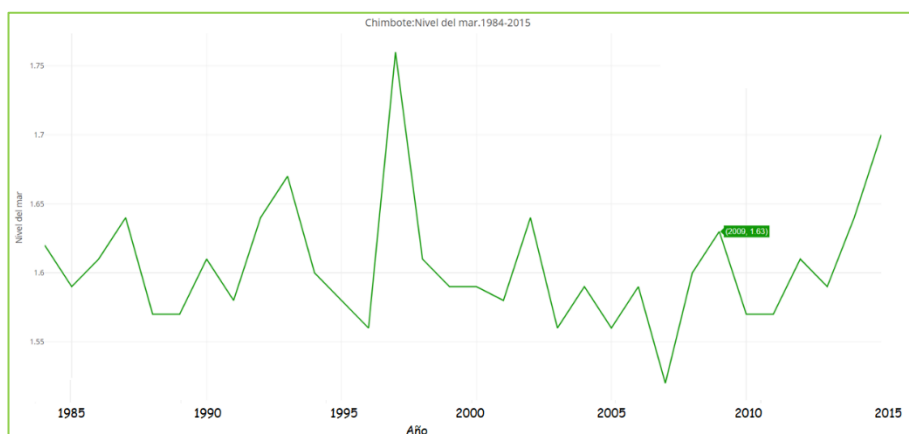
Figura 4A. Dinámica del nivel superficial del mar en la estación de Chimbote.
