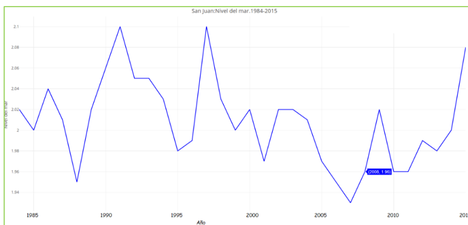
Figura 5A. Dinámica del nivel superficial del mar en la estación de San Juan.
