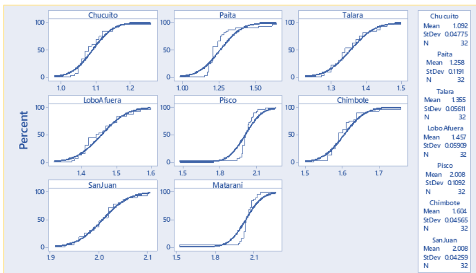
Figura 8A. Función de distribución de probabilidad (CDF) del nivel superficial del mar de las estaciones de Chucuito, Paita, Talara, Lobos de Afuera, Pisco Chimbote, San Juan y Matarani. 1984-2015.
