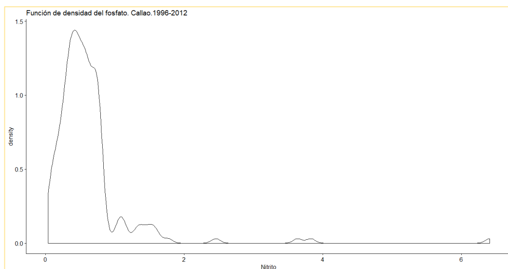
Figura 25A. Función de densidad empírica de la variable nitrito.
