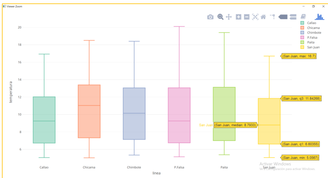
Figura 54. Boxplot de la temperatura en las líneas de monitoreo: Callao, Chicama, Chimbote, P. Falsa, Paíta y San Juan.
