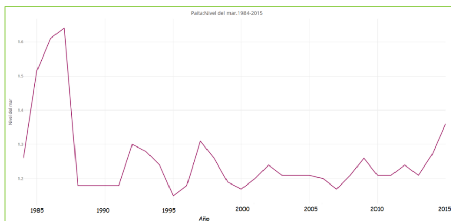
Figura 2A. Dinámica del nivel superficial del mar en la estación de Paita.
