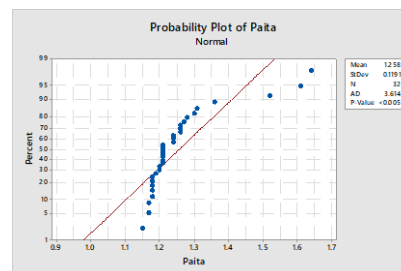
(b) Gráfico de probabilidad normal del Nivel superficial del mar de la estación de Paíta. 1984-2015.
