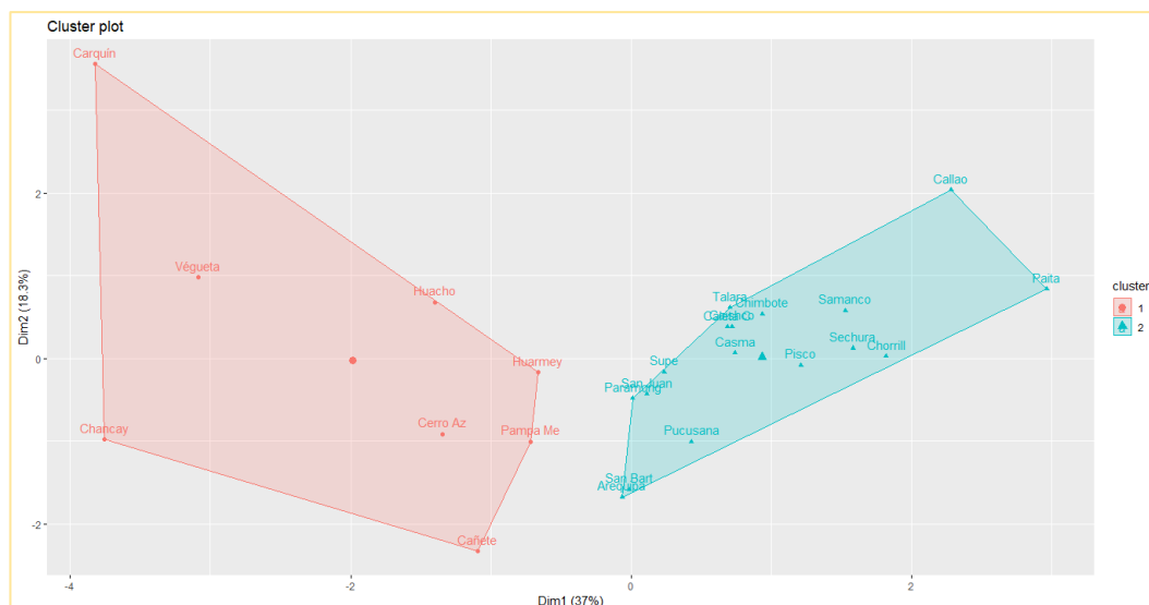
Figura 37. Agrupación robusta del pH de las 25 zonas de monitoreo
