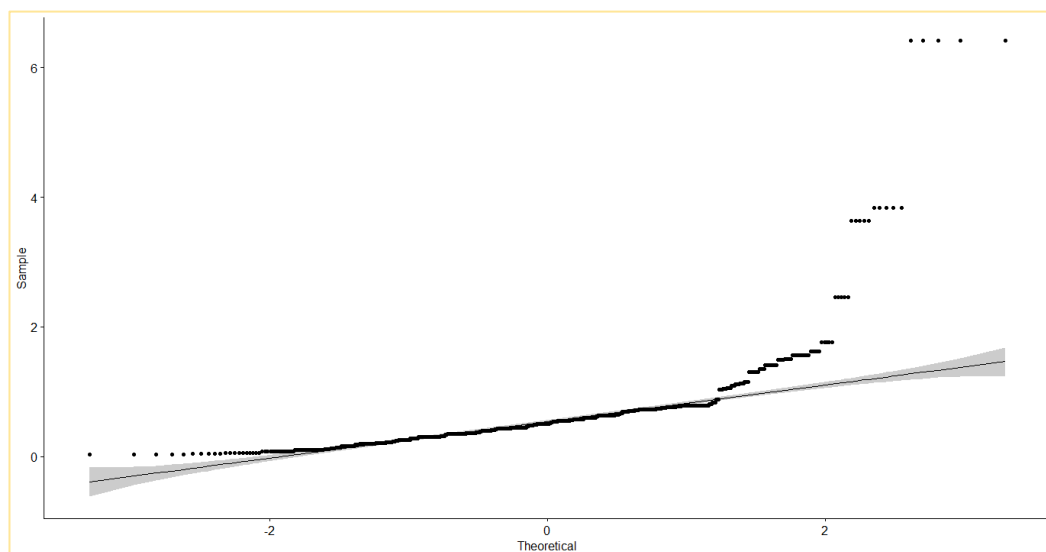
Figura 26A Q-Q plot de la variable nitrito.
