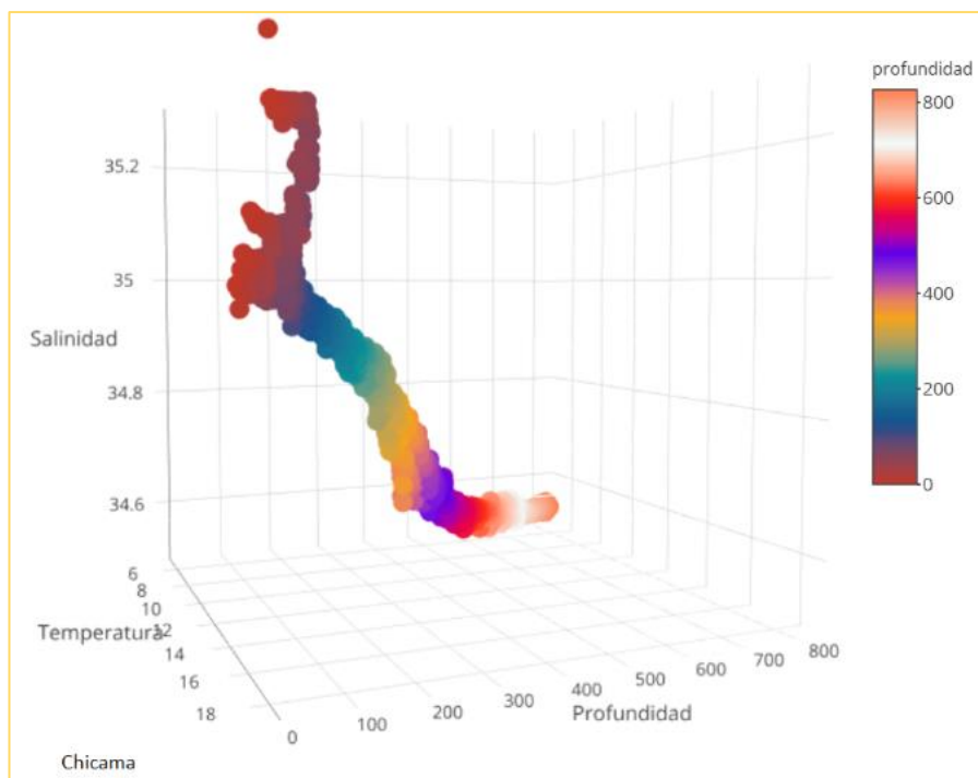
Figura 49A. Distribución conjunta de la temperatura y salinidad de acuerdo la profundidad de medición en Chicama. file:///D:/00TESIS.DOCTORADO.2017.2018/GRAFICOS%20R%2011NOV2018/PROFUNDIDATEMPSALCHICAMA.html
