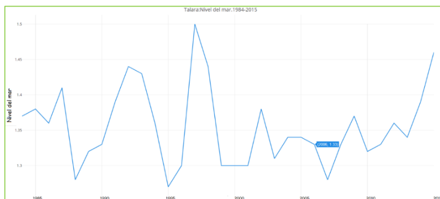
Figura 1A. Dinámica del nivel superficial del mar en la estación de Talara.
