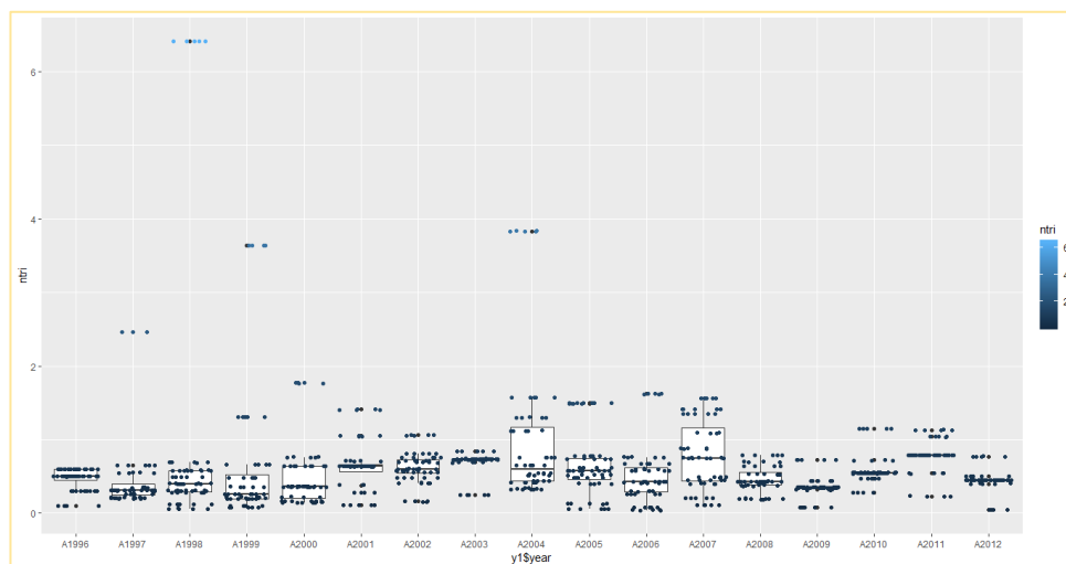
Figura 26A. Evolución anual del nitrito:1996-2012.
