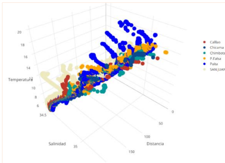
Figura 41A Distribución conjunta de la temperatura y salinidad de acuerdo la distancia de medición en la líneas de Callao, Chicama, Chimbote, Punta Falsa, Paíta y San Juan.
