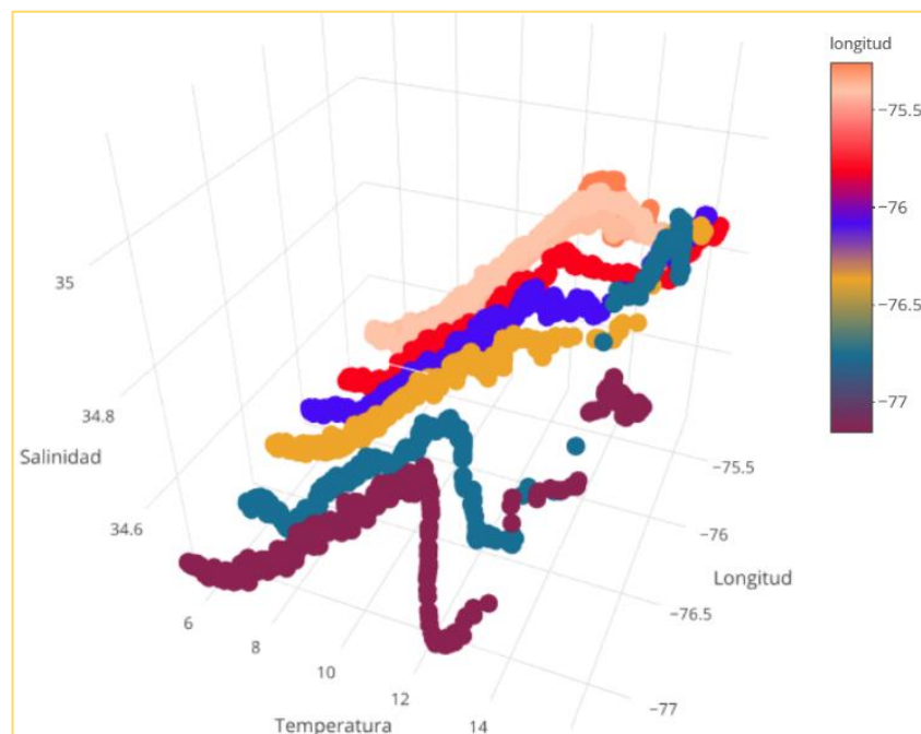
Figura 58A. Distribución conjunta de la temperatura y salinidad de acuerdo con la longitud en San Juan.
