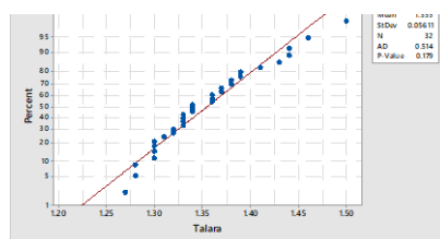
(c) Gráfico de probabilidad normal del Nivel superficial del mar de la estación de Talara. 1984-2015.
