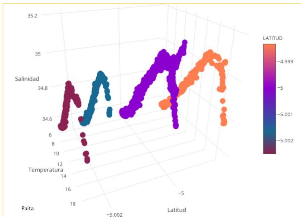
Figura 54A. Distribución conjunta de la temperatura y salinidad de acuerdo con la latitud en Paita.
