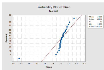
(e) Gráfico de probabilidad normal del Nivel superficial del mar de la estación de Pisco. 1984-2015.
